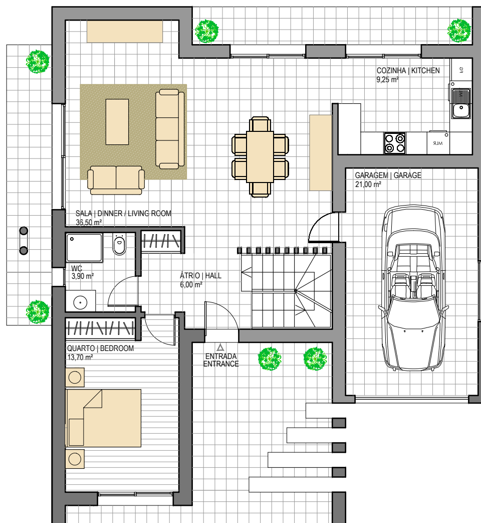
PLANTA PISO 0
