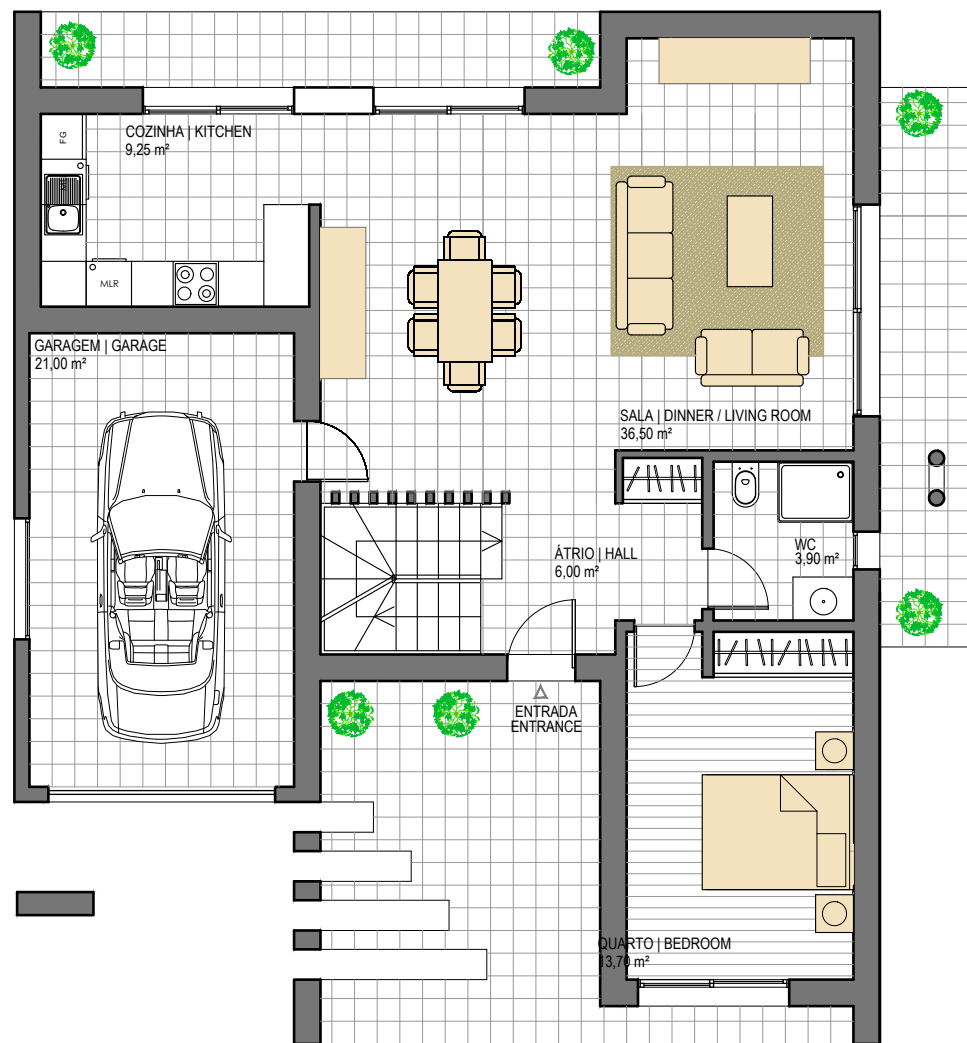
PLANTA PISO 0
