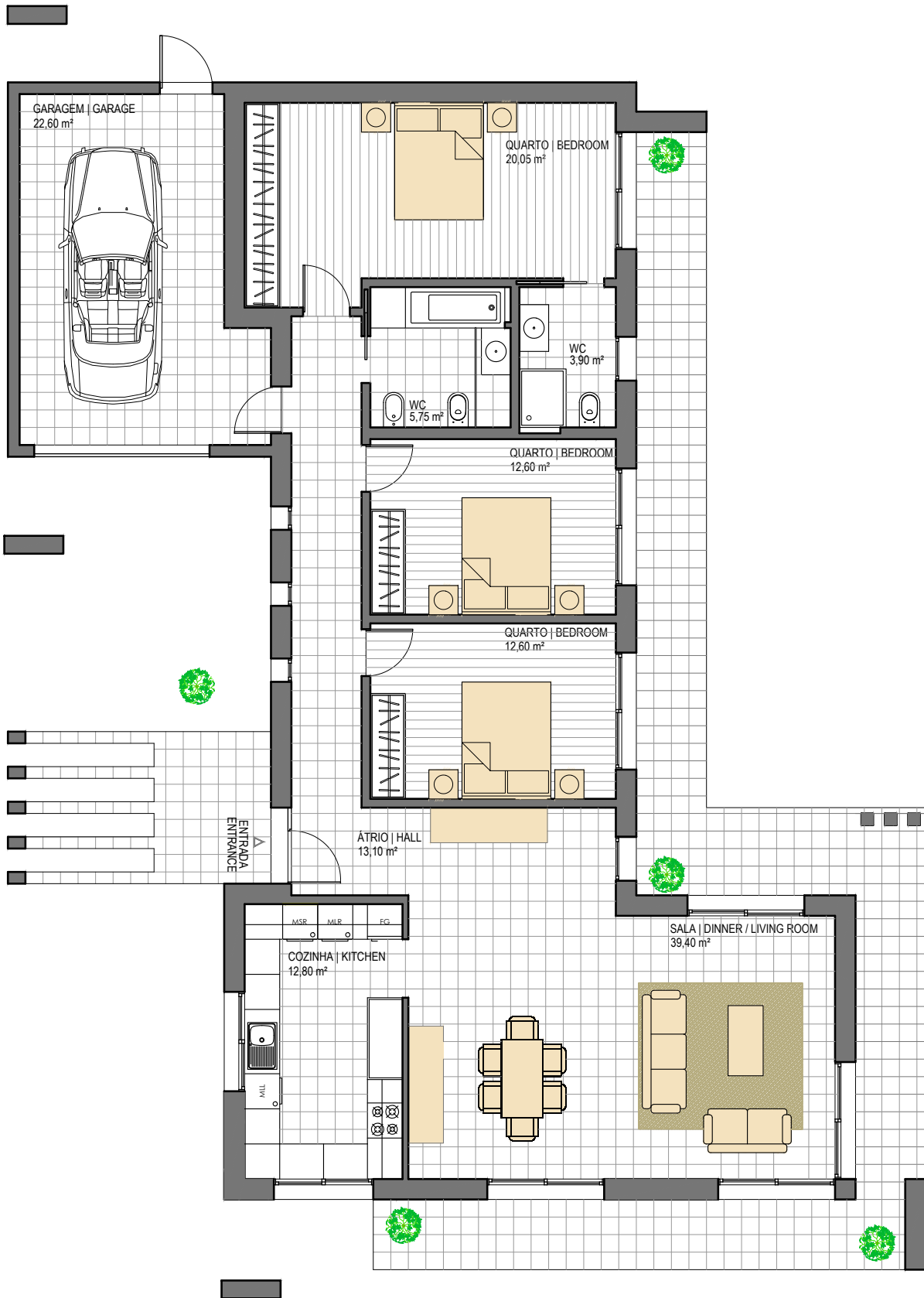
PLANTA PISO 0
