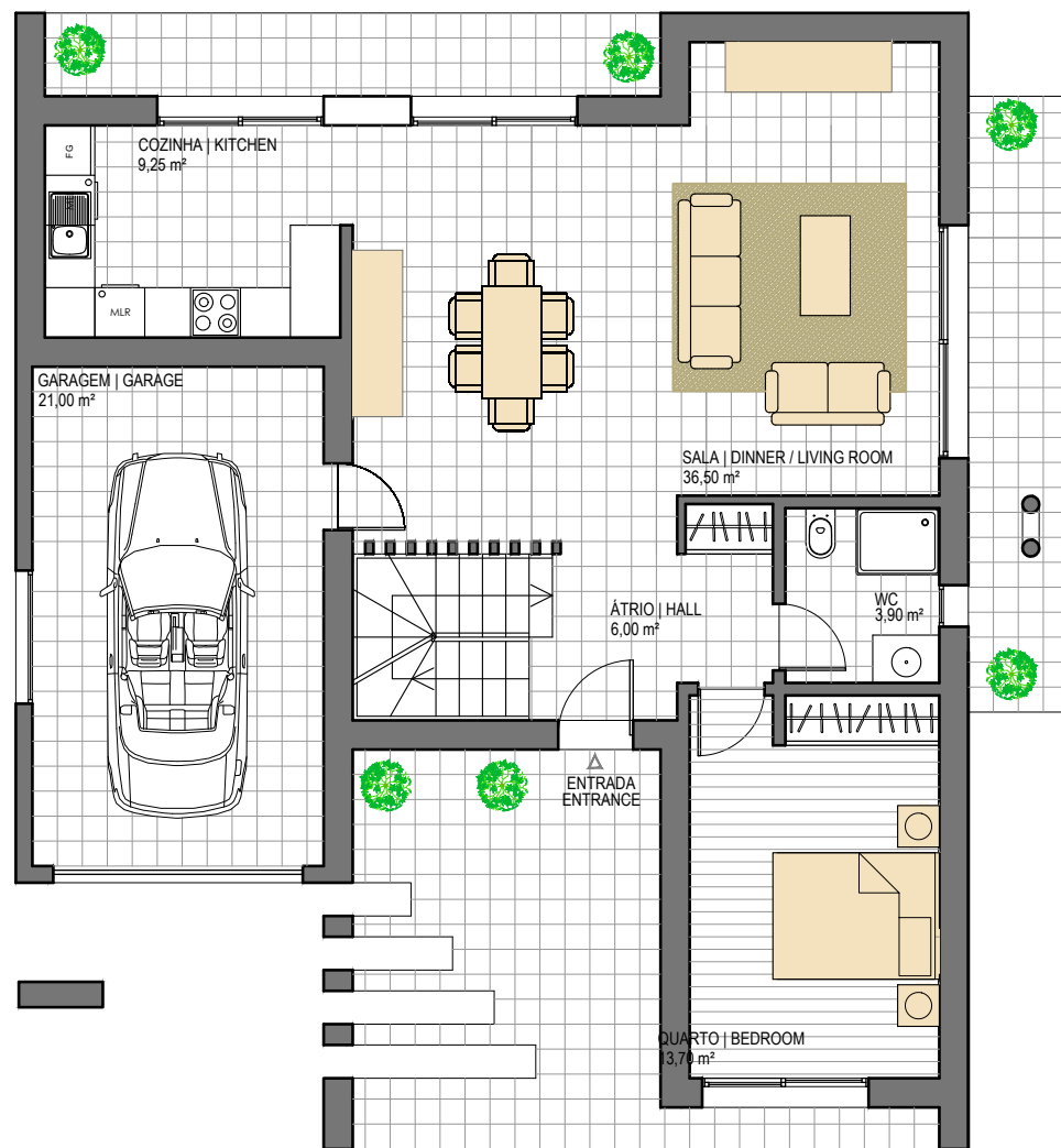
PLANTA PISO 0
